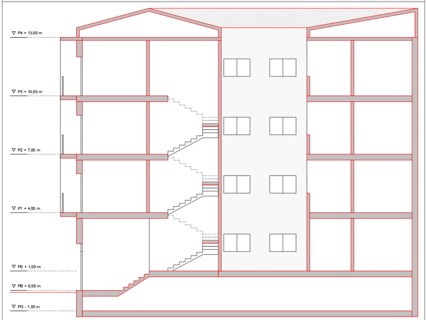
Croquis de la sección 1:
